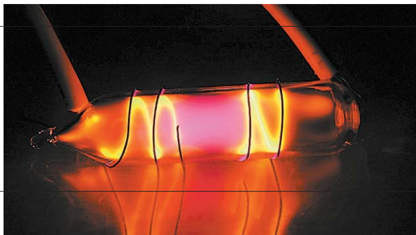
В разряде неон светится оранжевым.
