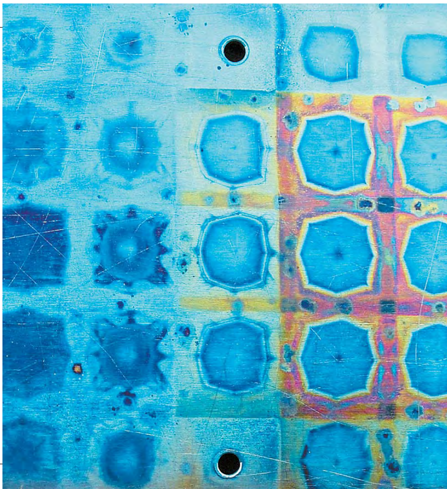
Титановая пластина из магниторазрядного насоса; цвета — результат интерференции в пленках соединений титана и остаточных газов.
