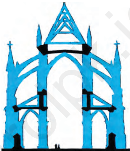
Схема готичного храму в розрізі
